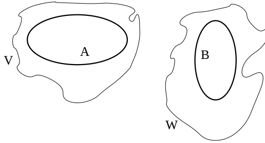
Непересекающиеся окрестности замкнутых множеств
