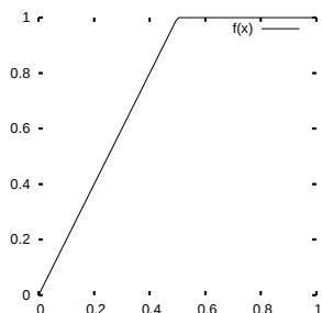
График функции \phi_1(t)
