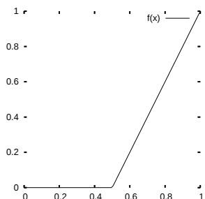
График функции \phi_0(t)
