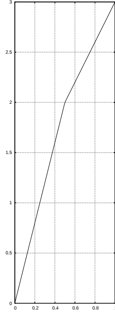
График функции \psi_2(t)
